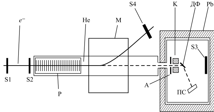
Рис. 5. Схема эксперимента [70]: P — многослойная структура (1000 слоев полиэтилена); S — сцинтилляционные детекторы; M — магнит; A — детектор антисовпадений; K — коллиматор; ДФ — дифракционный кристалл; PC — пропорциональный счетчик; Pb — свинцовая защита
