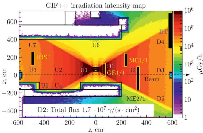
Рис. 3. Карта интенсивности радиационного поля источника ^{137}\text{Cs} установки GIF++ [11]. Указаны позиции детекторов, расположенных в зоне облучения (CSC, DT, RPC и GEM)
