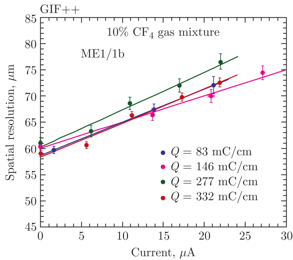
Рис. 4. Пространственное разрешение камеры ME1/1b, полученное в мюонном пучке на установке GIF++, в зависимости от средней величины тока в субкамере. Q — величина накопленного заряда (мКл/см)
