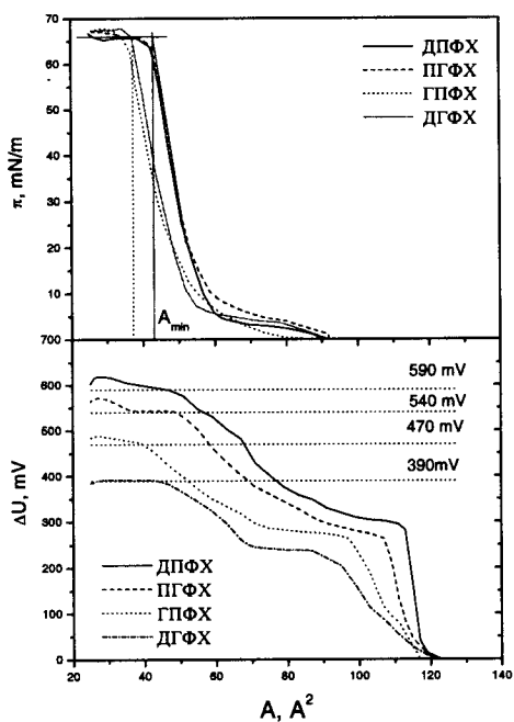
Рисунок 3. ( \pi - A ) и ( \Delta V - A ) изотермы и для липидных монослоев из ДПФХ (—), ПГФХ (----), ГПФХ (---) и ДГФХ (-·-·-).
