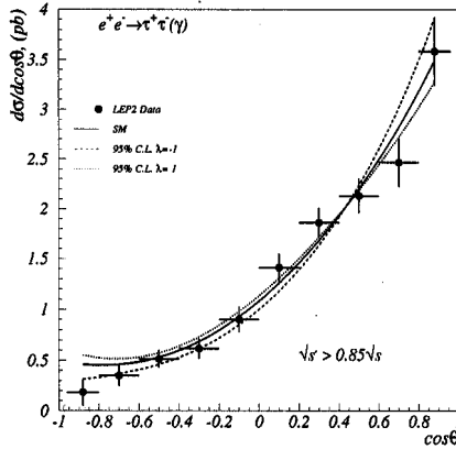
Рис. 3: Угловые распределения процессов e^+e^- \rightarrow \mu^+\mu^-(\gamma) (вверху) и e^+e^- \rightarrow \tau^+\tau^-(\gamma) (внизу), усредненные для данных, полученных при энергии столкновений 183-207 ГэВ. Линиями показаны предсказания Стандартной Модели, вычисленные для средней по интегральной светимости энергии соударений \sqrt{s} = 195.3 ГэВ, а также предсказания модели с дополнительными субмиллиметровыми пространственными измерениями, вычисленные при значениях массового параметра теории струн M_s , равных полученным пределам s для \lambda = -1 и \lambda = +1 .
