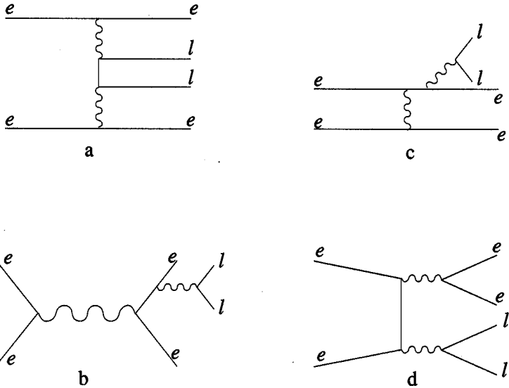
Рис. 1: Диаграммы, дающие вклад в процесс e^+e^- \rightarrow e^+e^-l^+l^- ( l = e, \mu, \tau ). а - мультипериферическая диаграмма, б - аннигиляция, с - тормозное излучение, д - конверсия.
