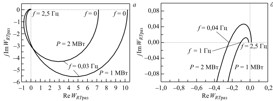
Рис. 9. Амплитудно-фазовые частотные характеристики разомкнутой системы (а) и их фрагменты (б) при средней мощности 1 и 2 МВт с расходом натрия через активную зону 78 м 3 /ч
