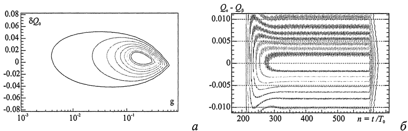
Рис. 3. Карты: (а) изолиний \alpha(g, \delta Q_0) = \alpha_l [4] и (б) изоамплитуд a_e(n, Q_e - Q_\beta) = a_l [5]
