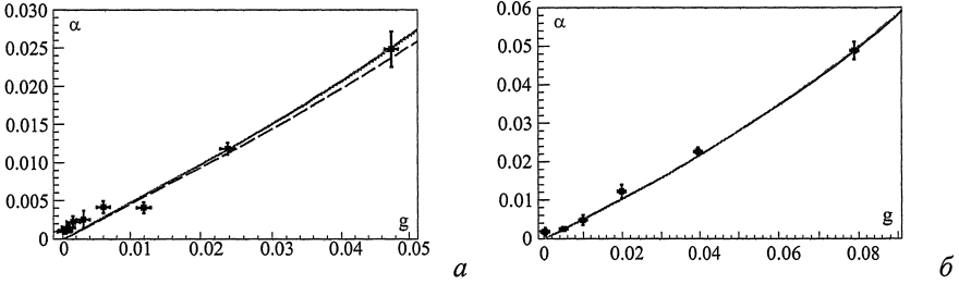
Рис. 2. Расчетные декременты затухания и результаты измерений горизонтальных (а) и вертикальных (б) когерентных поперечных колебаний пучка протонов с энергией 3.5 ТэВ в ЛНС [5, 15]
