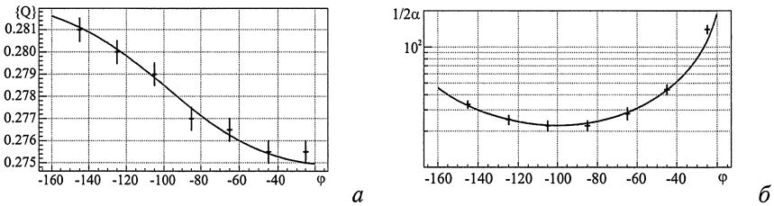
Рис. 4. Расчетные зависимости величины \{Q\} (а) и коэффициента резонансного усиления (б) от фазового параметра \varphi фильтра Гильберта (сплошные линии) в сопоставлении с результатами экспериментальных измерений [7]
