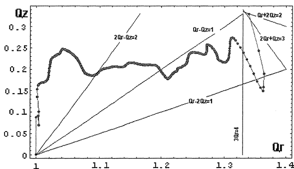
Рис. 1. Диаграмма рабочей точки циклотрона С235
