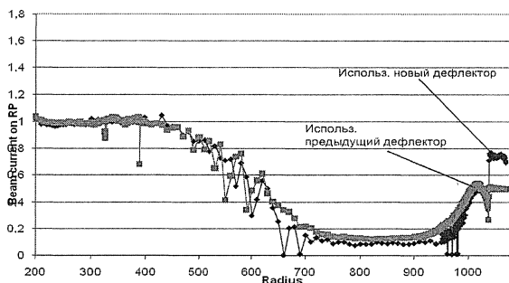
Рис. 3. Зависимость измеренной интенсивности тока пучка (нормирована на величину тока на радиусе 300мм) от радиуса в циклотроне С235 при использовании дефлекторов нового и предыдущего типов
