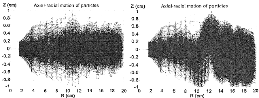
Рис. 8. Вертикальное движение пучка с начальным эмиттансом \varepsilon_z = 200 \mu , начиная от ионного источника. Слева – нет B_r , внизу – есть B_r типа в средней плоскости
