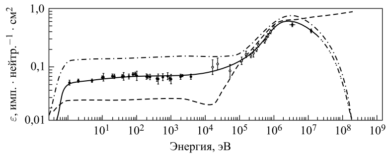
Рис. 3. ЭЗЧ счетчика СНМ-14 с комбинированным замедлителем
