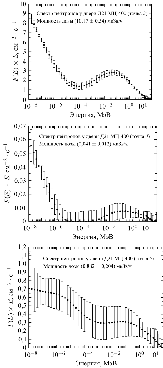
Рис. 5. Спектры нейтронов в точках 2, 3 и 5 на МЦ-400
