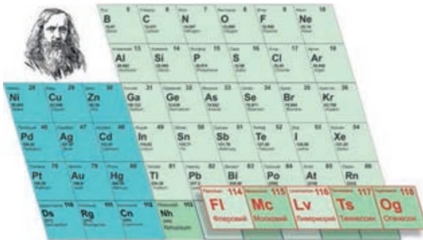
Часть Периодической таблицы элементов Д. И. Менделеева
