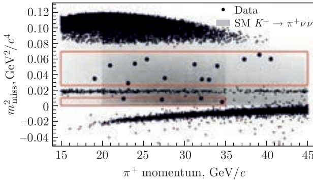
События-кандидаты в сверхредкий распад (в рамке) и фоновые события в переменных измеренного импульса заряженного пиона и квадрата недостающей массы, связанной с нейтрино
