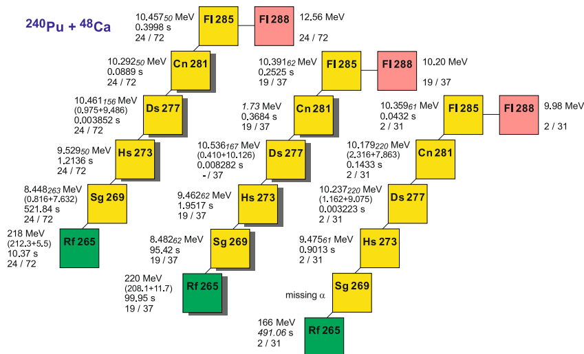
Новые цепочки распада ядра ^{285}\text{Fl}
