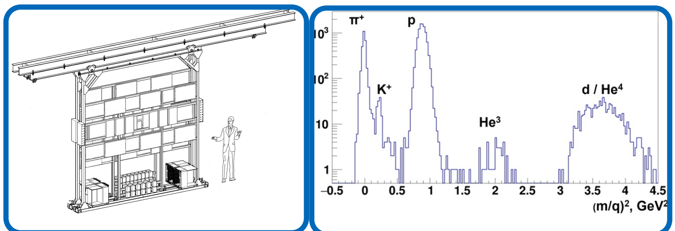
Рис. 10. Эскиз детектора TOF700 (слева) и результаты идентификации заряженных частиц по времени пролета в TOF700 (справа). Fig. 10. Schematic drawing of TOF700 (left) and the results of identification of charged particles by TOF700 (right).
