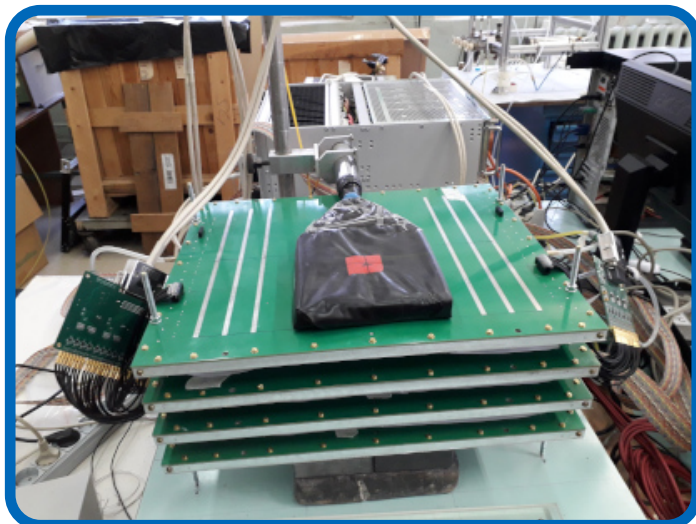
Рис. 12. Изготовленные камеры MRPC (фото слева) для предлагаемой конструкции время-пролетной системы TOF SPD (рисунок справа).
