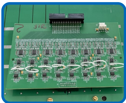
Рис. 13. Плата электроники считывания данных с камер MRPC.
