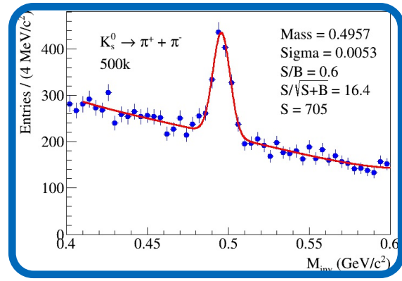
Рис. 6. Сигналы \Lambda -гиперонов и K_S^0 -мезонов в спектрах эффективных масс (p, \pi^-) и (\pi^+, \pi^-) . Fig. 6. Signals of \Lambda -hyperons and K_S^0 mesons in the effective mass spectra of (p, \pi^-) and (\pi^+, \pi^-) .
