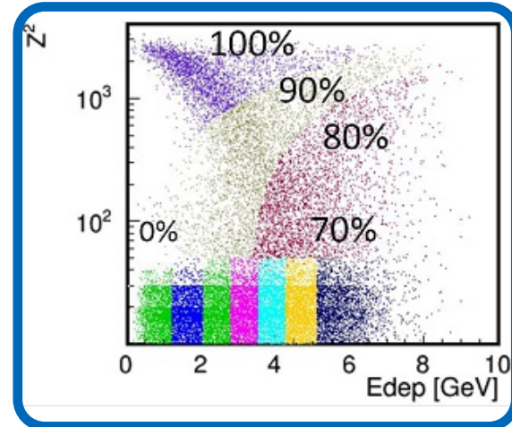
Рис. 7. Слева: Идентификация заряженных \pi^-, \pi^+, K^+ мезонов, протонов, дейтронов, тритонов во времяпролетной системе. Справа: классы центральности событий, определенные по амплитуде в годоскопе фрагментов ( Z^2 ) и энергии, выделенной в переднем адронном калориметре ( E_{dep} ).
