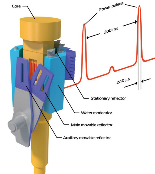
Схематическое изображение работы реактора ИБР-2
