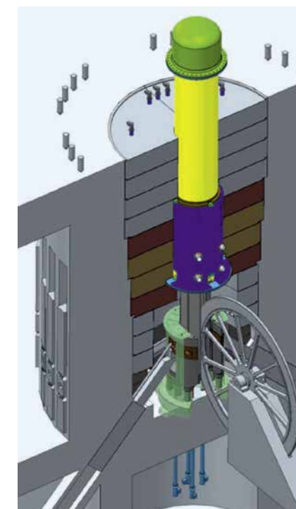
Схематическое изображение Импульсного реактора 4-го поколения
