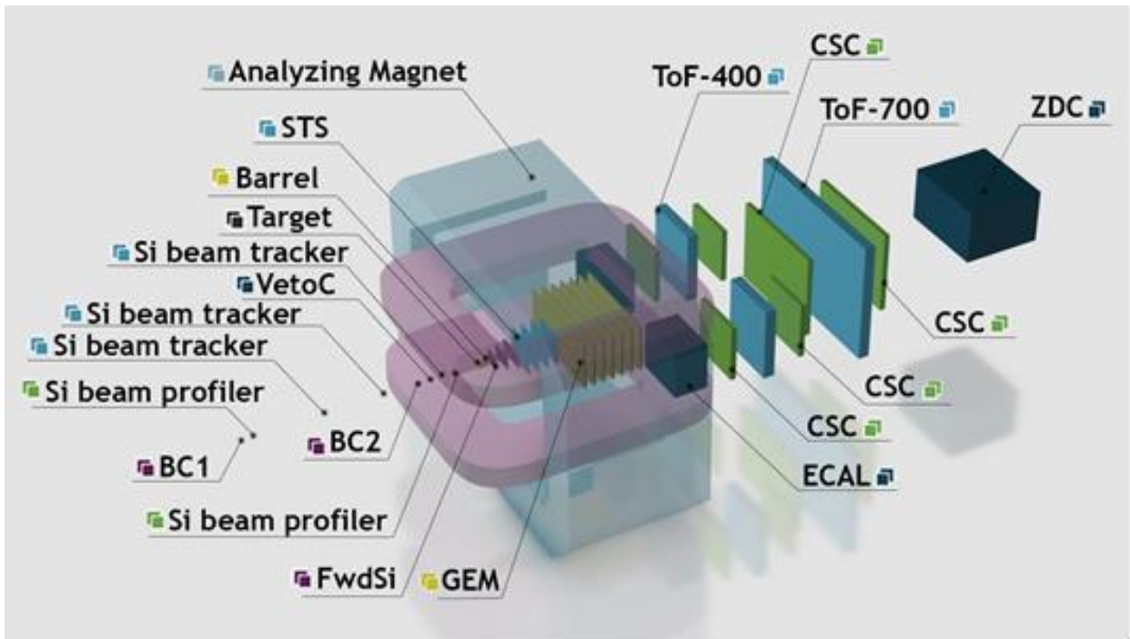
Рис. 3. Полная конфигурация детекторов BM@N для реализации программы исследований в пучках тяжелых ионов
