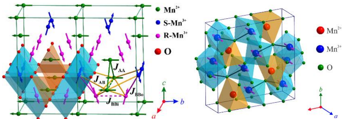
Рис. 25. Индуцированный давлением колоссальный рост температуры магнитного упорядочения в геометрически фрустрированном оксиде Mn_3O_4
