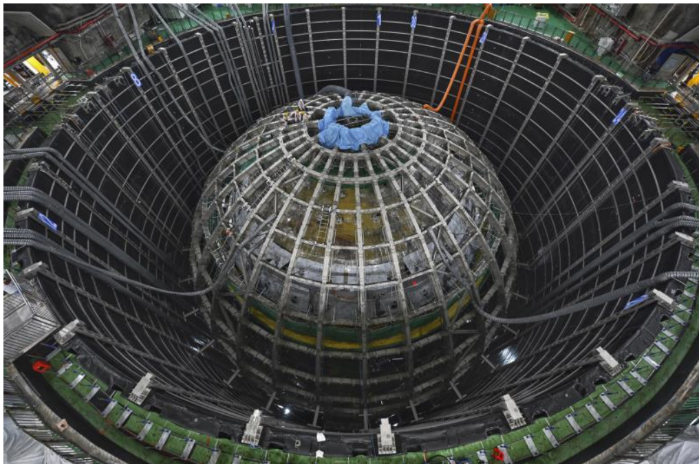
Рис. 16. Текущее состояние сборки детектора JUNO
