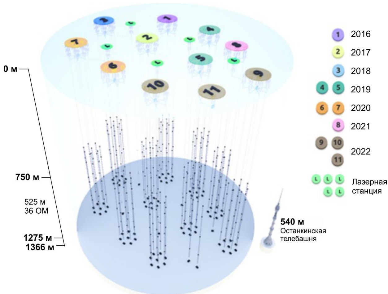
Рис. 10. Статус развертывания телескопа по состоянию на конец 2022 года. Установка содержит 2916 оптических модулей и семь лазерных калибровочных источников света на пяти станциях
