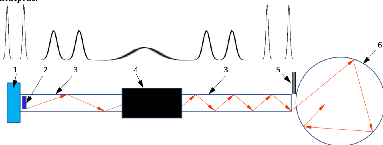
Рис. 24. Идея источника УХН для импульсного источника с использованием временной фокусировки. 1 – замедлитель, 2 – конвертер УХН, 3 – зеркальный нейтронвод, 4 – фокусирующее устройство, 5 – быстрый затвор, 6 – ловушка УХН
