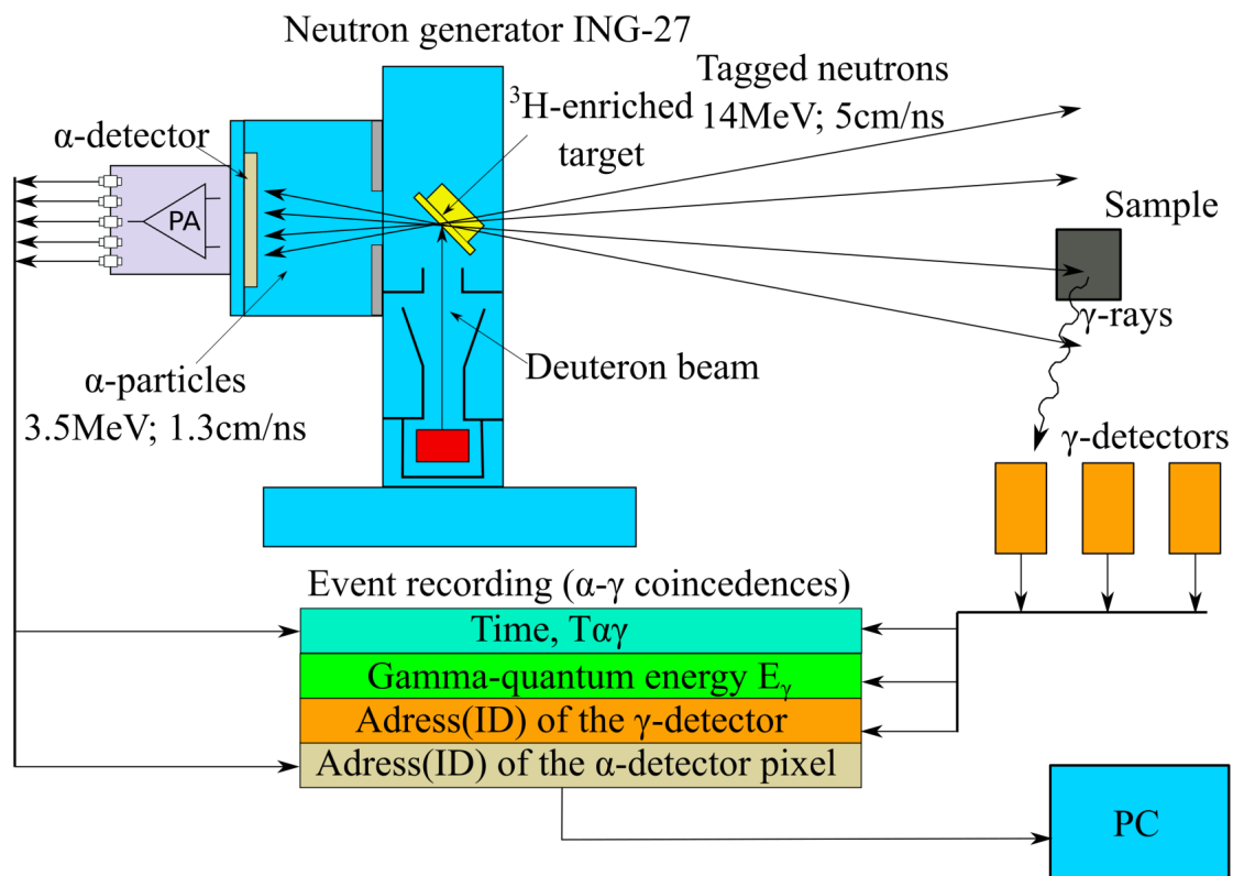
Рис. 23. Схема экспериментов с использованием метода меченых нейтронов для изучения взаимодействия быстрых нейтронов с ядрами
