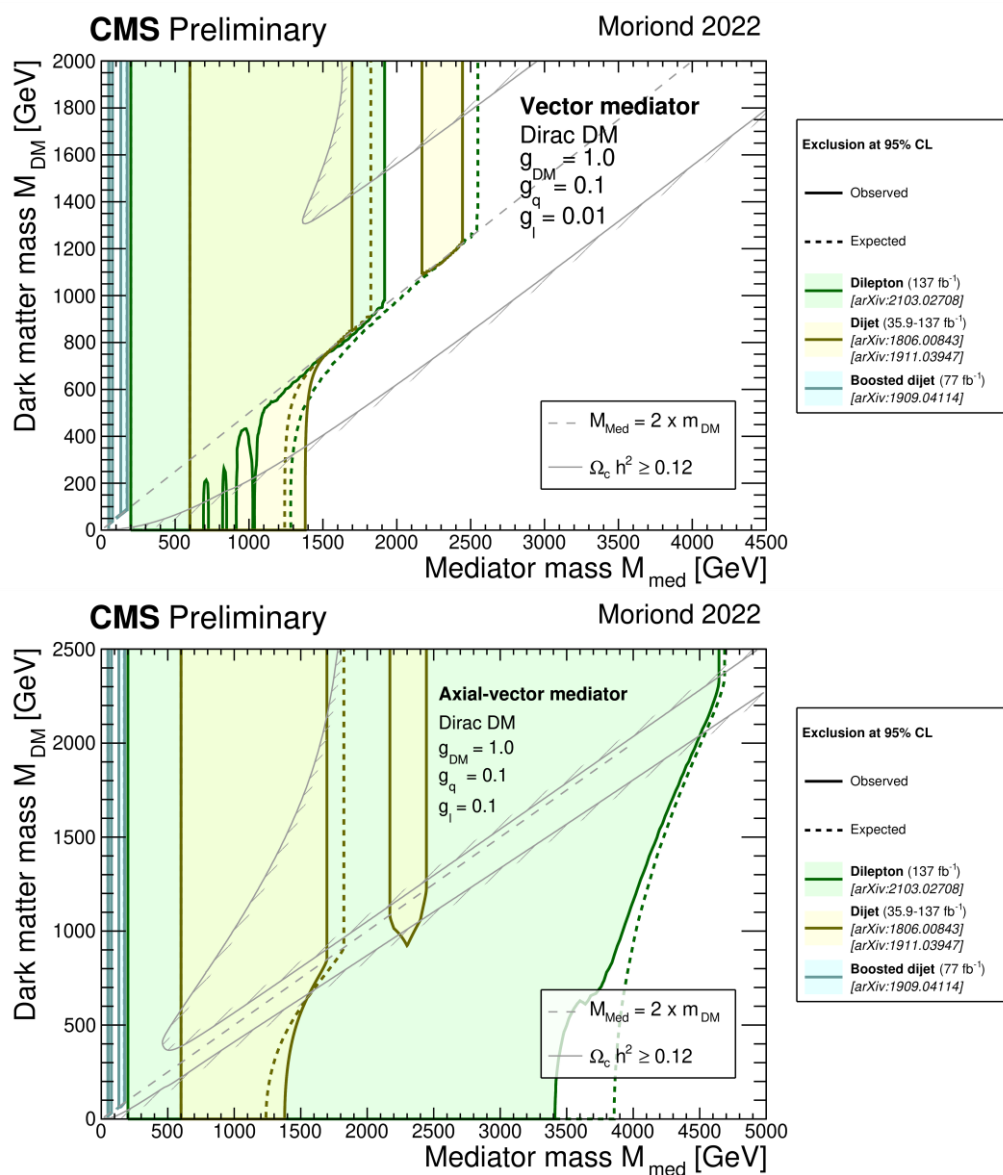
Рис. 15. В объединенном канале рождения пары струй и пары лептонов в событиях, зарегистрированных в эксперименте CMS на LHC, определены пределы (95% С.Л.) на массы частиц-кандидатов на роль частиц темной материи m_{DM} и частицы-переносчика взаимодействия с темным сектором M_{med} . Закрашенная область соответствует закрытым значениям масс для векторного (вверху) и псевдовекторного (внизу) переносчика
