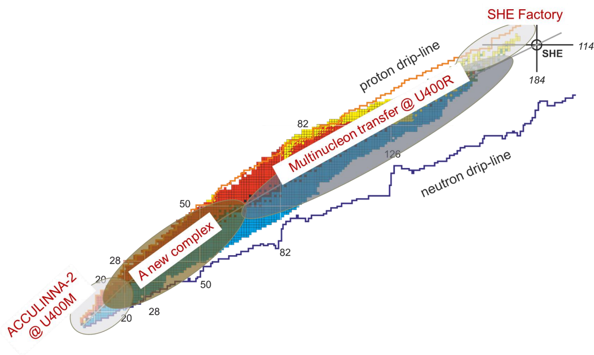
Рис. 20. Способы получения ядер в разных областях карты ядер, развиваемые в ЛЯР
