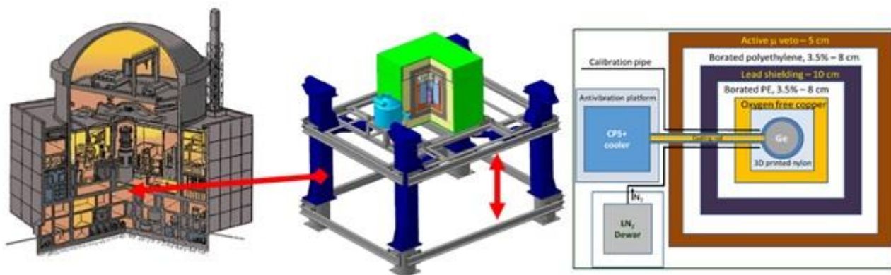
Рис. 18. Схема установки \nu GeN, нацеленной на детектирование CEvNS. Установка расположена непосредственно под реактором #3 КАЭС (слева), на специальном подъемном устройстве (в центре), позволяющем изменять поток антинейтрино в HPGe-детекторе, окруженном комплексной активной и пассивной защитой (справа)
