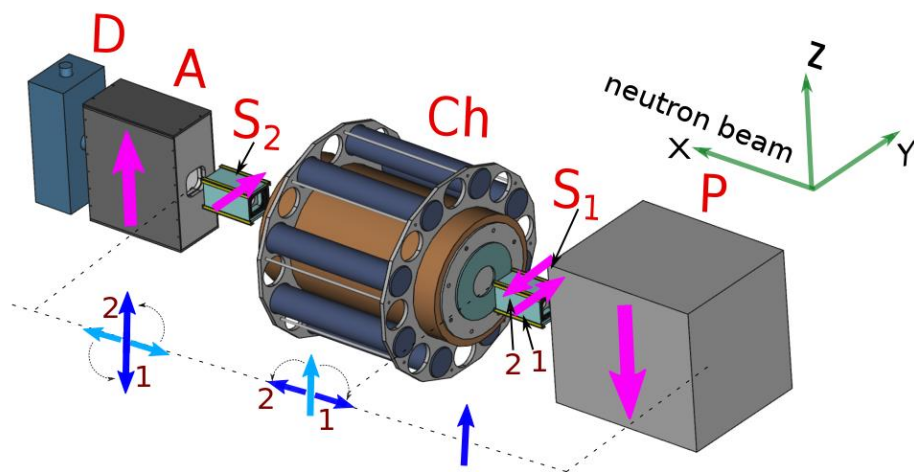
Рис. 22. Схема эксперимента для измерения T-нечетных эффектов в делении. P – SEOP поляризатор; Ch – камера деления, окруженная гамма-детекторами; A – анализатор; D – детектор нейтронов; S1, S2 – устройства управления спином. Розовые стрелки на рисунке указывают направление магнитного поля, синие стрелки – направление спина нейтрона
