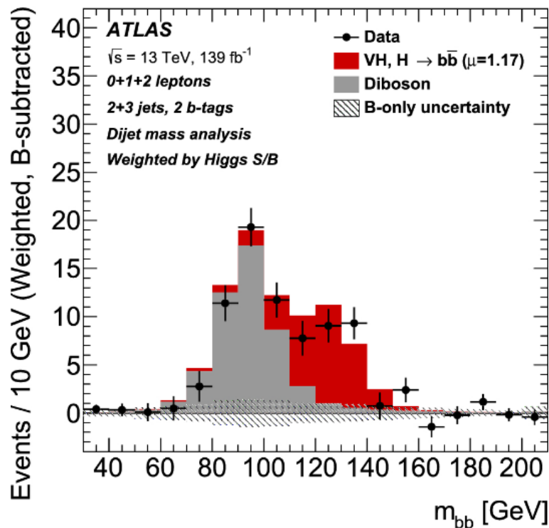
Рис. 14. Полученное в pp -взаимодействиях при энергии 13 ТэВ в эксперименте ATLAS распределение по инвариантной массе двух b -струй в процессах ассоциированного рождения бозона Хиггса с W - и Z -бозонами и его распадом на два b -кварка. Вычтен вклад всех фоновых процессов, за исключением двухбозонных – WZ и ZZ
