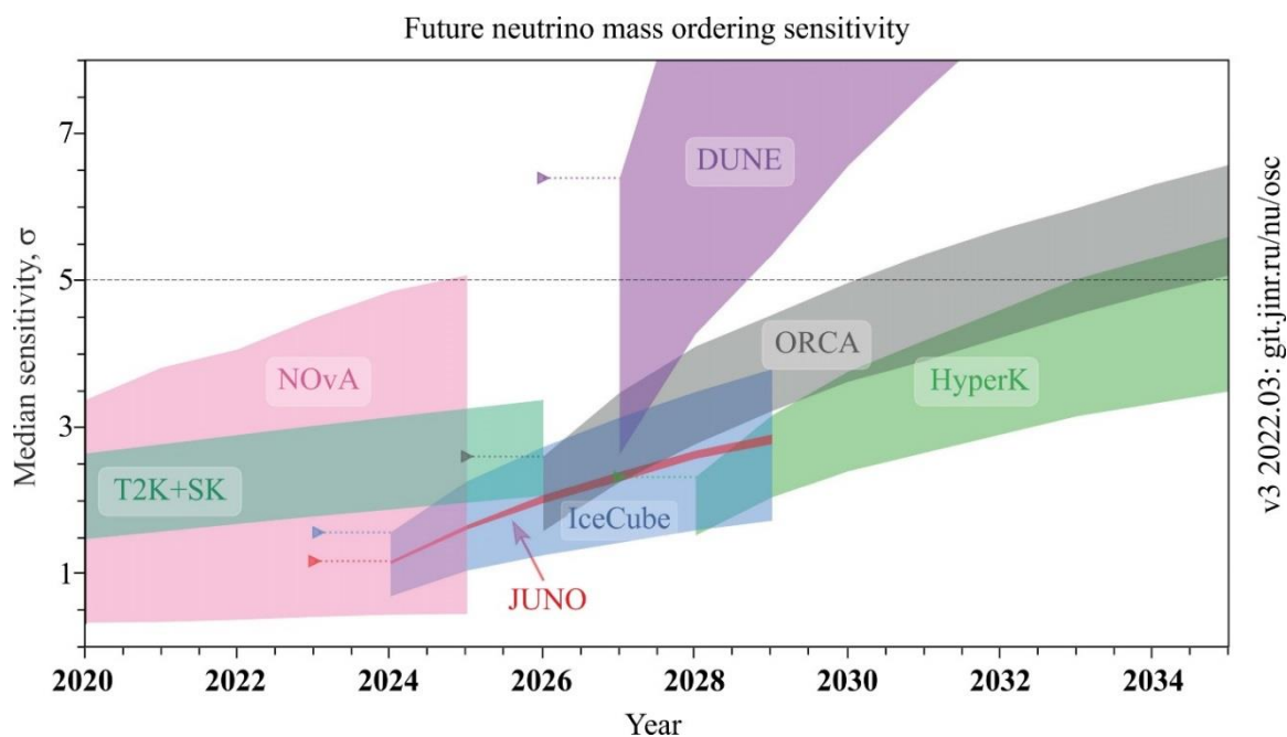
Рис. 17. Чувствительность к иерархии масс нейтрино действующих и планируемых экспериментов. Полосы представляют собой весь диапазон возможных измерений в зависимости от остальных параметров
