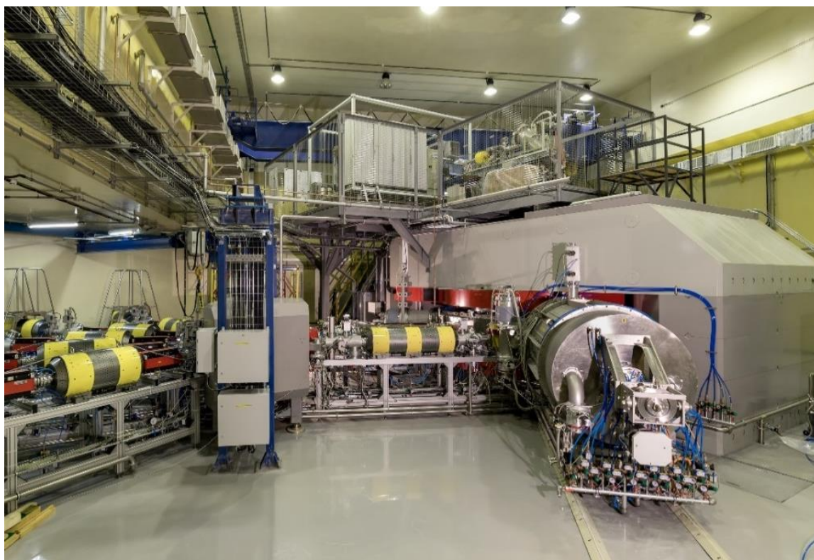
Рис. 19. Циклотрон ДЦ-280 Фабрики СТЭ
